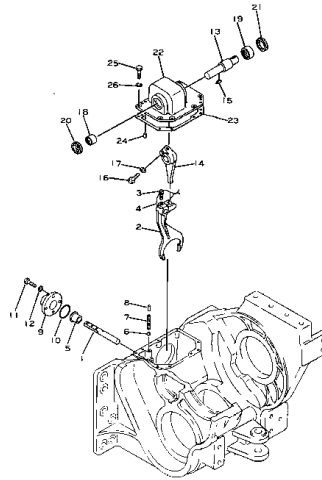
シフトフォーク およびカバー Fig. 106 SHIFT FORK AND COVER (1/2)
