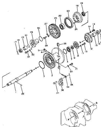
Fig. 104 ギヤー および ワイヤ ドラム GEAR AND WIRE DRUM
