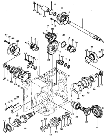
P.T.O. シフトおよびギヤー 適用年 2001 - FIG. 102A P.T.O. SHAFT AND GEAR (D30 SERIAL NO. 2001 -)
