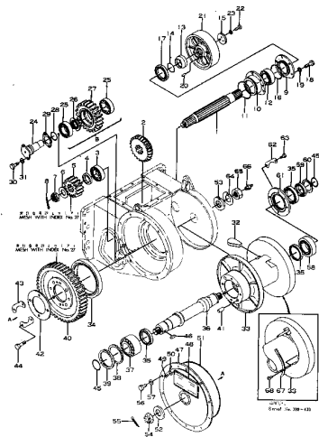
ギヤ・ドラム ドラム 適用機種 FIG. 103 GEAR AND DRUM (D30 SERIAL NO. (300) - (4999))
