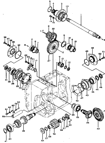
P.T.O. シフト 歯およびギヤー 適用 機種 FIG. 102 P.T.O. SHAFT AND GEAR (D30 SERIAL NO. (300) - (4999))
