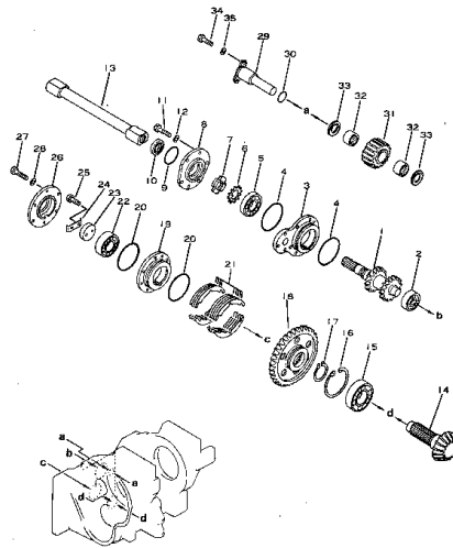
シャフトおよびギヤ Fig. 102 P.T.O. SHAFT AND GEAR
