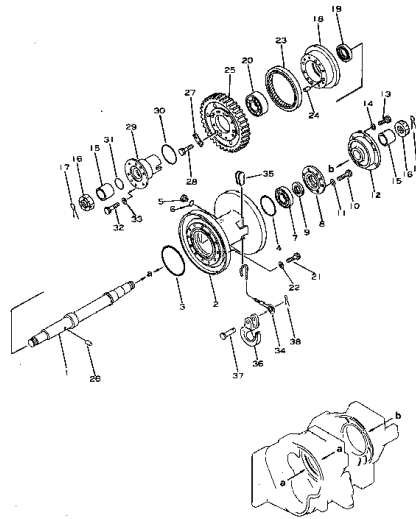
ギヤー および ワイヤ ドラム Fig. 104 GEAR AND WIRE DRUM
