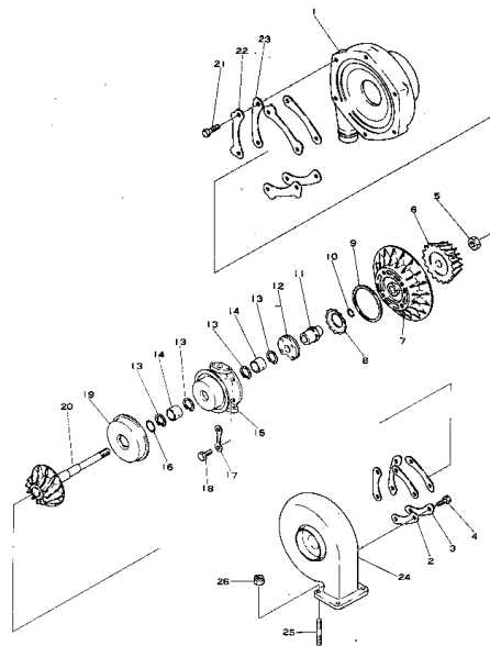
ターボチャージャー Fig.103 TURBOCHARGER
