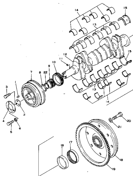
クランクシャフト、バイブレーションダンパーおよびフライホイール Fig. 204 CRANKSHAFT, VIBRATION DAMPER AND FLYWHEEL
