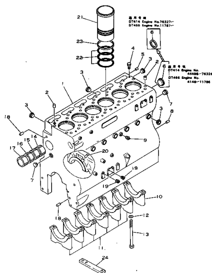
シリンダブロック Fig. 201 CYLINDER BLOCK
