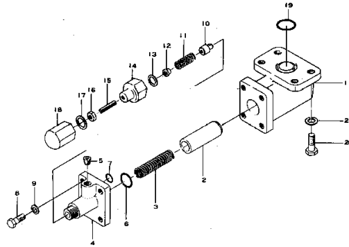
リリーフバルブ FIG. 113 RELIEF VALVE (適用号機 (Serial No. D (6001~9999))
