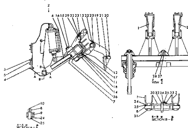
リッパシャング、ビーム、リンク Fig. 101 RIPPER SHANK, BEAM AND LINK (適用機種 (Serial No. D50A(5861)-(15400))
