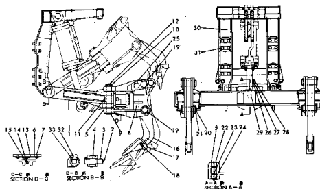
リッパ シャンク ビーム および リンク Fig. 102 RIPPER SHANK, BEAM AND LINK (適用号数 (Serial No. D50S (5861)~(15400)))
