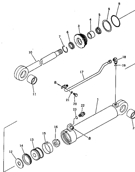
ハイドロリック シリンダ Fig. 211 HYDRAULIC CYLINDER
