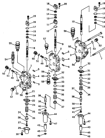
パイドロリクコントロールバルブ Fig. 234 HYDRAULIC CONTROL VALVE(1/2) (D31S Serial No. 1001~)
