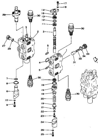
Fig. 136 HYDRAULIC CONTROL VALVE(2/3) (適用機種 D31ASerial No. 2001～)
