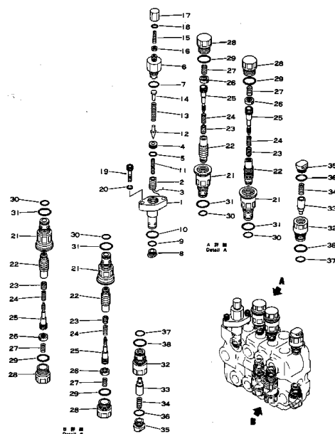
Fig. 137 ハイドロリック コントロール バルブ HYDRAULIC CONTROL VALVE (3/3) (D31A Serial No. 2001-(28000))
