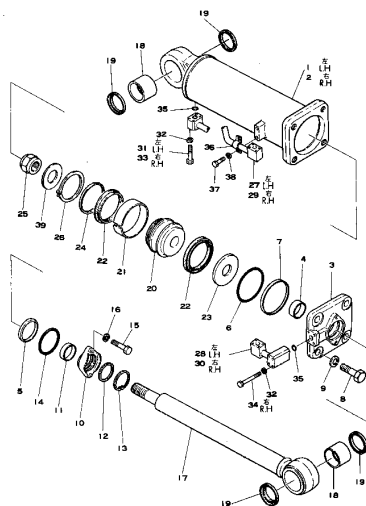
リフトシリンダ (適用機種 1010～1296) Fig. 211 LIFT CYLINDER (Serial No. 1010～1296)
