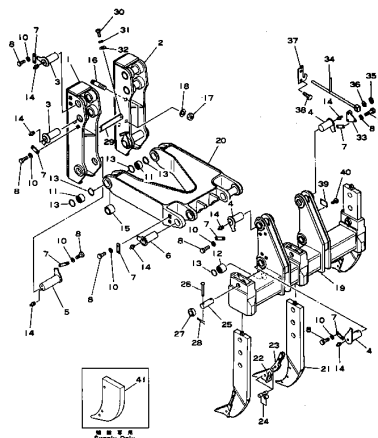
リッパ シェンク、ビームおよびリンク (適用機種 1010~1631) Fig. 201 RIPPER SHANK, BEAM AND LINK (Serial No. 1010~1631)
