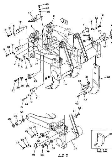
リッパシャング、ビームおよびリンク (適用 専用) Fig. 201B RIPPER SHANK, BEAM AND LINK (Serial No. 4001 ~)
