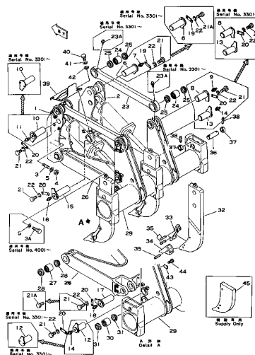
リッパ シェンク、ビームおよびリンク (適用機種) Fig. 201A RIPPER SHANK, BEAM AND LINK (Serial No. 1632~4000)
