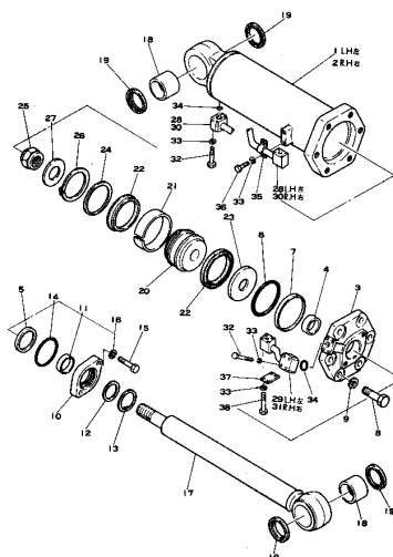
リフトシリンダ (適用機種) Fig. 211A LIFT CYLINDER (Serial No. 1297~3299)
