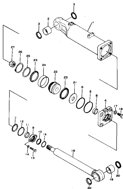
Fig.111 リッパ シリンダ (適用号機 1010~1296) RIPPER CYLINDER (Serial No. 1010~1296)
