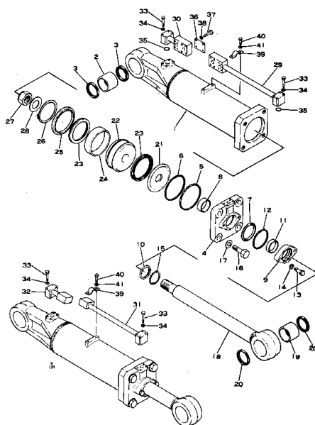
Fig. 111A リッパ シリンダ (適用号機 Serial No. 1297~3299)
