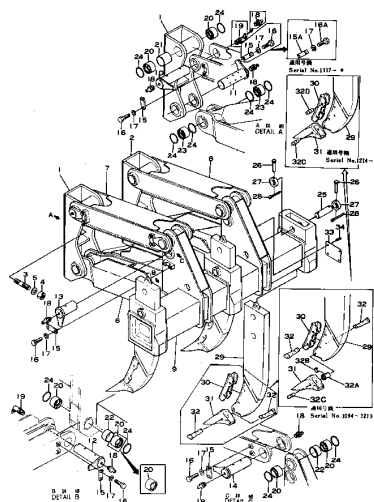
Fig.101 リッパ シェンク、ビームおよびリンク RIPPER SHANK, BEAM AND LINK (適用機番 Serial No. 1010~1631)
