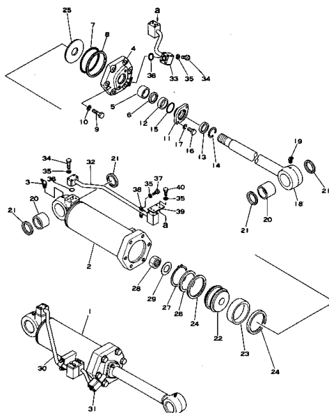
リフトシリンダ (適用機種) Fig. 211A LIFT CYLINDER (D150 Serial No. 8421~8476) (D155 Serial No. 17001~19775)
