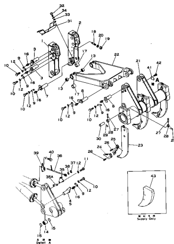
リッパ シャック、ビームおよびリンク (適用機種 D150 Serial No. 8140 ~ 8328) Fig. 201 RIPPER SHANK, BEAM AND LINK (D155 Serial No. 8651 ~ 10262)
