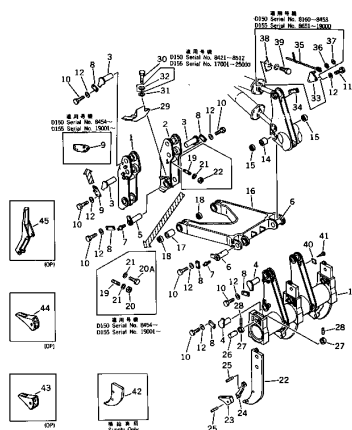
リッパ ショック、ビームおよびリンク (D150 Serial No. 8421~) Fig. 201B RIPPER SHANK, BEAM AND LINK (D150 Serial No. 8421~) (D155 Serial No. 17001~)
