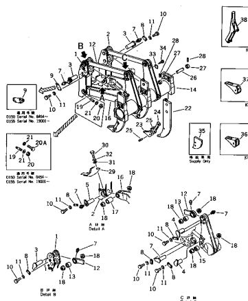
リッパ シャング、ビームおよびリンク (適用 号 機) Fig. 101B RIPPER SHANK, BEAM AND LINK (D150 Serial No. 8421~) (D155 Serial No. 17001~)
