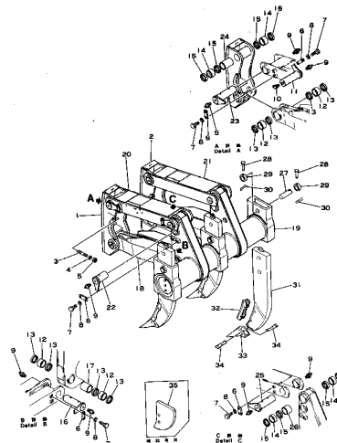
Fig. 101 リッパ シャフト、ビームおよびリンク RIPPER SHANK, BEAM AND LINK (D150 Serial No. 5508~8328) (D155 Serial No. 5508~10262)
