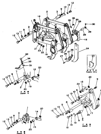
Fig. 101A リッパシャック、ビームおよびリンク RIPPER SHANK, BEAM AND LINK (D150 Serial No. 8329~8420) (D155 Serial No. 10263~17000)
