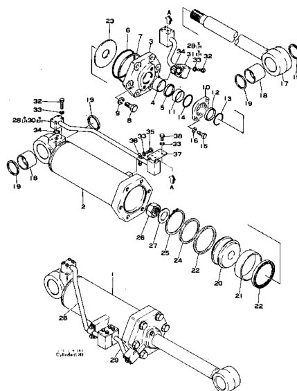
リフトシリンダ (適用機種) Fig. 111A LIFT CYLINDER (D150 Serial No. 8329~8420) (D155 Serial No. 10263~17000)
