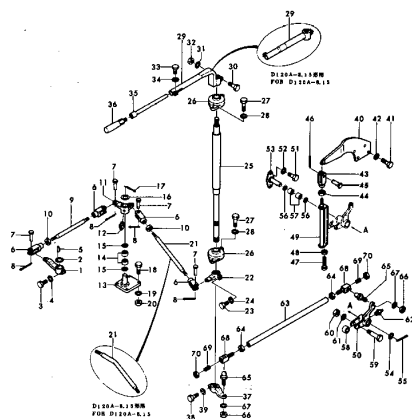
FIG. 108 コントロールレバーおよびキックアウト CONTROL LEVER AND KICKOUT (Hydraulic Type, D120A-8,15,18 AND D125A-18)
