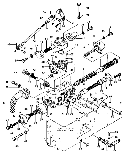
FIG. 1-04 コントロールバルブ CONTROL VALVE (ケーブル式) (Cable Type, D120A-18 AND D125A-18)
