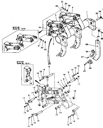
Fig.561 リッパシャフト、ビーム、及びリンク Fig.561 RIPPER SHANK, BEAM AND LINK
