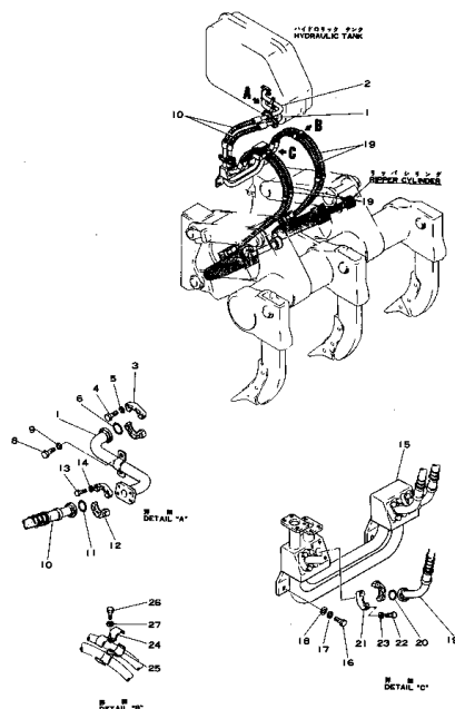
リッパパイピング Fig.562 RIPPER PIPING
