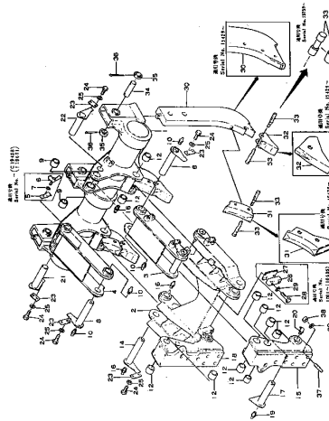
リッパ フレーム FIG. 101 RIPPER FRAME
