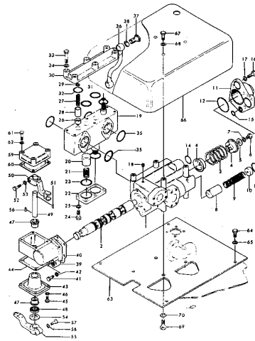
コントロールバルブ FIG. 109 CONTROL VALVE (D80-8)
