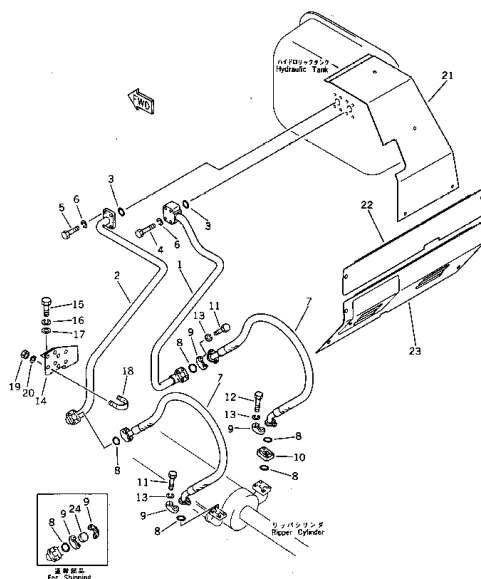
ハイドロリックパイピング Fig. 121 HYDRAULIC PIPING
