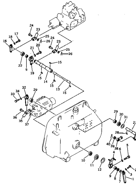
ハイドロリック タンク (D60-65S Serial No. 40001~) Fig. 137 HYDRAULIC TANK(3/3)
