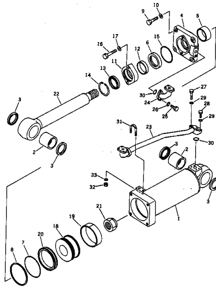
ハイドロリック シリンダ Fig. 111 HYDRAULIC CYLINDER
