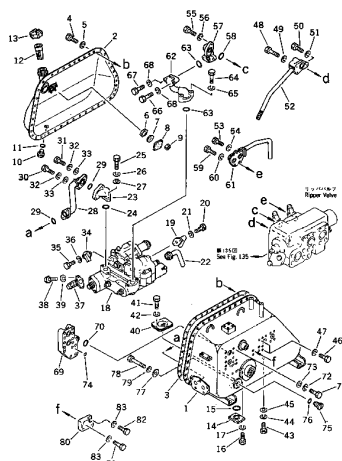
ハイドロリック タンク Fig. 131 HYDRAULIC TANK (1/2)
