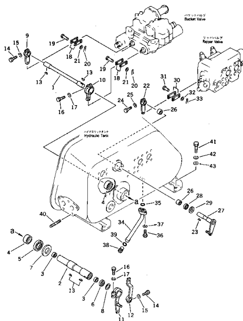
ハイドロリック タンク Fig. 132 HYDRAULIC TANK (2/2)
