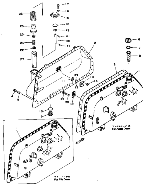
ハイドロリック タンク Fig. 131 HYDRAULIC TANK (1/2)
