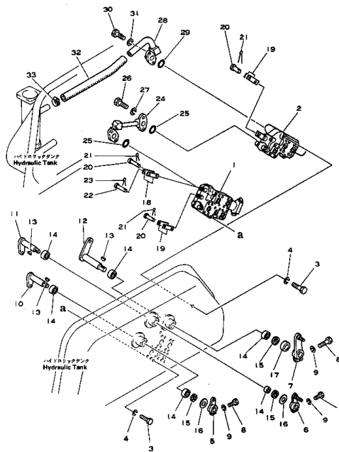
ハイドロリック タンク (チルトドーザー用) Fig. 133 HYDRAULIC TANK (2/2) (For Tilt Dozer)
