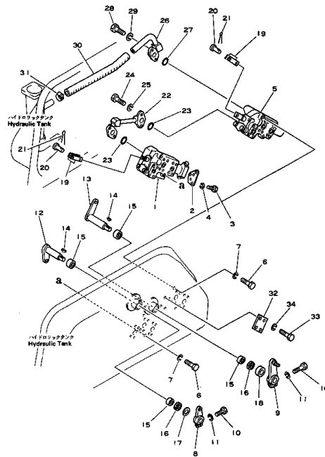
Fig. 132 HYDRAULIC TANK (2/2) (For Angle Dozer) ハイドロリック タンク (2/2) (アングルドーザ用)
