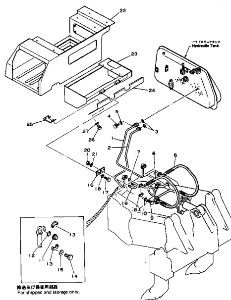
ハイドロリックパイピング Fig. 121 HYDRAULIC PIPING
