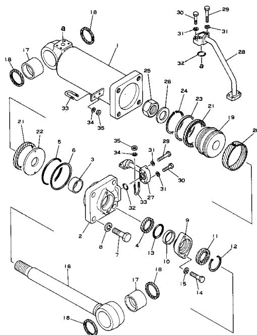
Fig. 111 シリンダ CYLINDER
