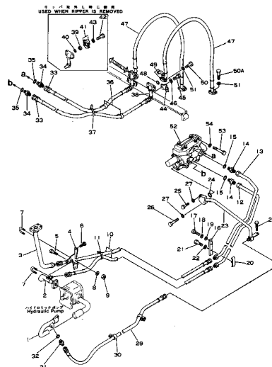
Fig. 121B ハイドロリックパイピング HYDRAULIC PIPING (D40,45A Serial No. (1801-))
