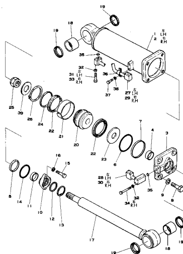
リフトシリンダ (適用機種 1010～1296) Fig. 211 LIFT CYLINDER (Serial No. 1010～1296)
