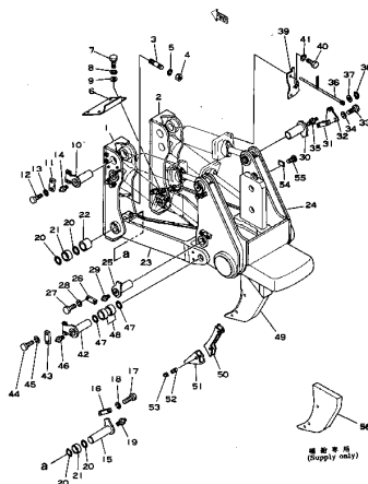
リッパ シャンク、ビームおよびリンク (適用号機 Fig. 201 RIPPER SHANK, BEAM AND LINK (Serial No. 1010 ~ 1631))
