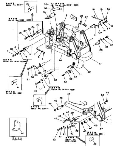
リッパ シャシ、ビームおよびリンク (適用 号 図) Fig. 201A RIPPER SHANK, BEAM AND LINK (Serial No. 1632-4000)
