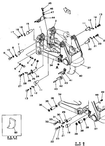
リッパ シャシ、ビームおよびリンク (適用 機種) Fig. 201B RIPPER SHANK, BEAM AND LINK (Serial No. 4001-)
