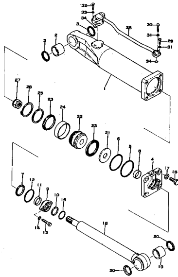
Fig. 111 リッパ シリンダ RIPPER CYLINDER
