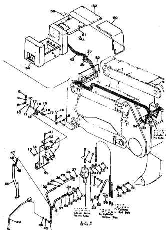
Fig. 135 ピン プラ - パイピング および コントロール レバー PIN PULLER PIPING AND CONTROL LEVER
