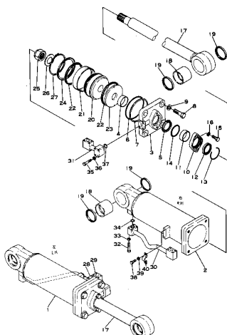
リフトシリンダ (適用機種) Fig. 211 LIFT CYLINDER (D150 Serial No. 6843~8159) (D155 Serial No. 6843~8650)
