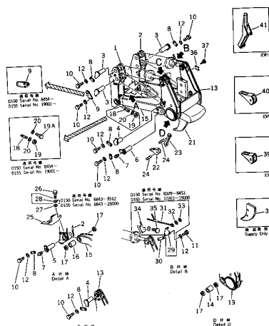
リッパ シャンク、ビームおよびリンク (D150 Serial No. 8421~) Fig. 201B RIPPER SHANK, BEAM AND LINK (D155 Serial No. 17001~)
