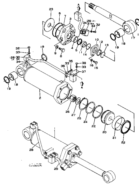
リフトシリンダ (適用号機) Fig. 211A LIFT CYLINDER (D150 Serial No. 8160~8420) (D155 Serial No. 8651~17000)
