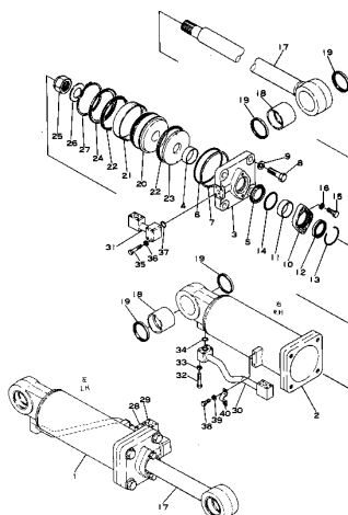
リフトシリンダ (適用機種: D150 Serial No. 6843~8159) Fig. 211 LIFT CYLINDER (D150 Serial No. 6843~8159) (D155 Serial No. 6843~8650)
