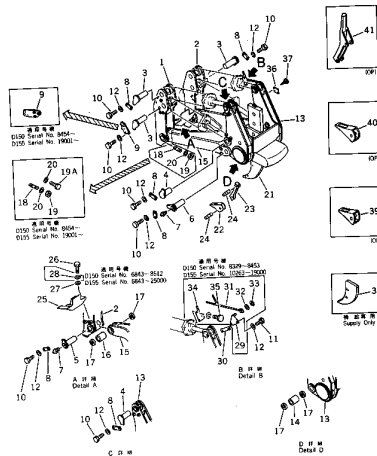
リッパ シャンク、ビームおよびリンク (適用機種 Fig. 201B RIPPER SHANK, BEAM AND LINK (D150 Serial No. 8421~) (D155 Serial No. 17001~))
