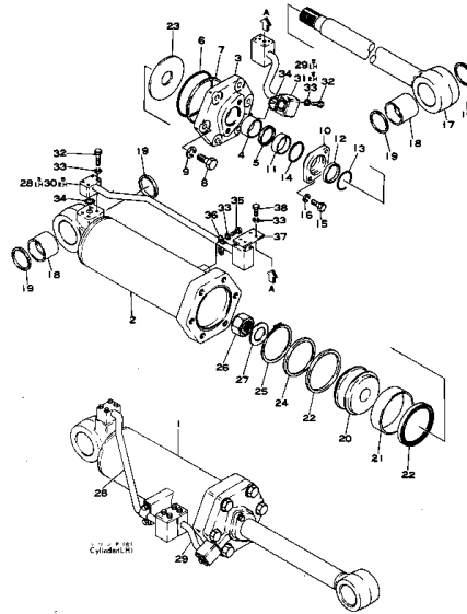
リフトシリンダ (適用機種) Fig. 111A LIFT CYLINDER (D150 Serial No. 8329~8420) (D155 Serial No. 10263~17000)
