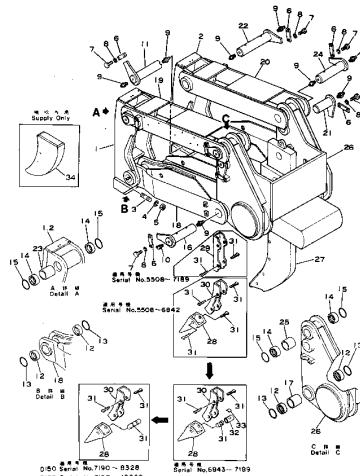
リッパ ショック、ビームおよびリンク Fig. 101 RIPPER SHANK, BEAM AND LINK (D150 Serial No. 5508-8328) (D155 Serial No. 5508-10262)
