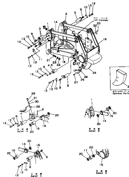
Fig. 101A リッパ シャンク、ビームおよびリンク RIPPER SHANK, BEAM AND LINK (D150 Serial No. 8329~8420) (D155 Serial No. 10263~17000)
