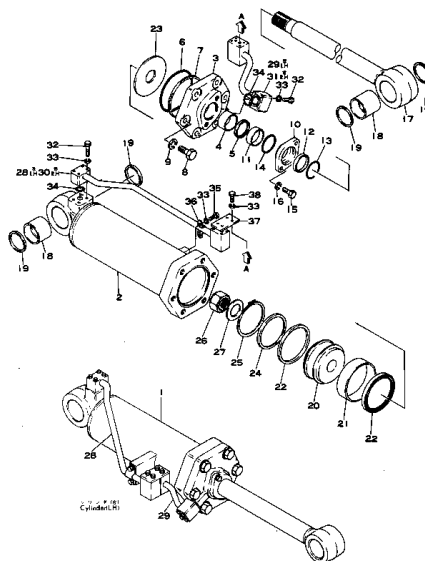
リフトシリンダ (D150 Serial No. 8329~8420) Fig. 111A LIFT CYLINDER (D155 Serial No. 10263~17000)
