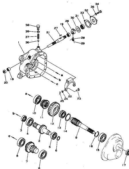
P.T.O. Fig. 106 P.T.O. (2/2)
