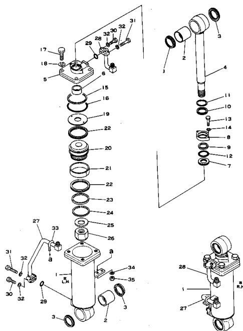
3 点 ヒッチ シリンダ Fig. 111 3-POINT HITCH CYLINDER
