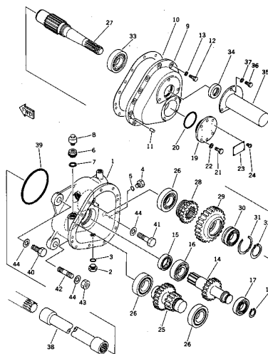
Fig. 205 P.T.O. (1/2)
