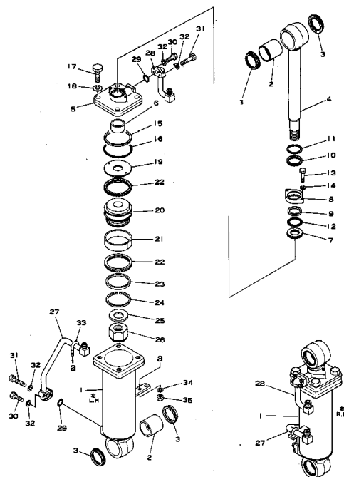
Fig. 1111 3点 ヒッチ シリンダ 3PT. HITCH CYLINDER
