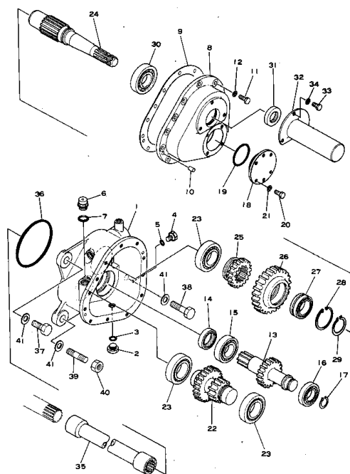
Fig. 1105 P.T.O. (1/2)
