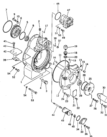
PTO ケース Fig. 205 P.T.O CASE
