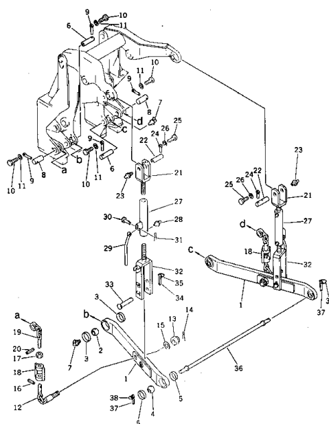
3 点 ヒッチ Fig. 202 3-POINT HITCH (2/2)
