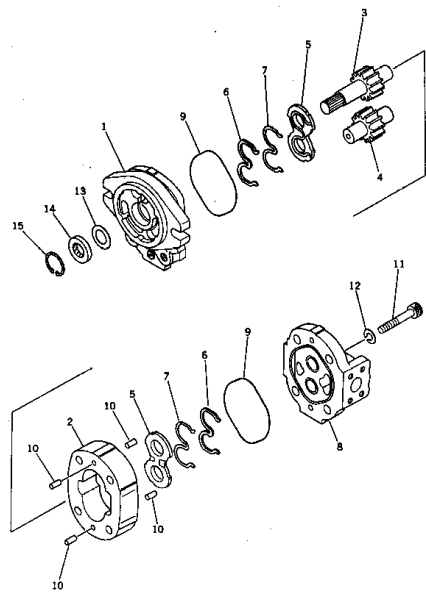
P.T.O. ポンプ Fig. 208 P.T.O. PUMP
