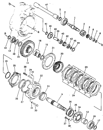
PTO シャフト 及び ギヤ Fig. 206 P.T.O SHAFT AND GEAR
