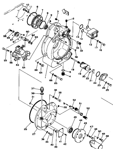
Fig. 105 P.T.O CASE
