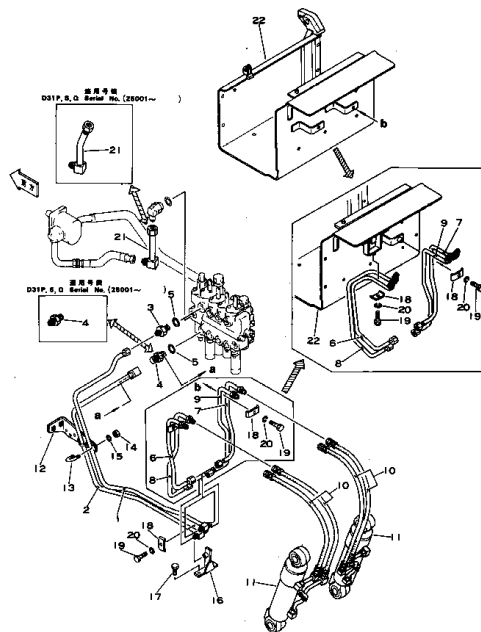
ハイドロリック オイルパイピング Fig. 121 HYDRAULIC OIL PIPING
