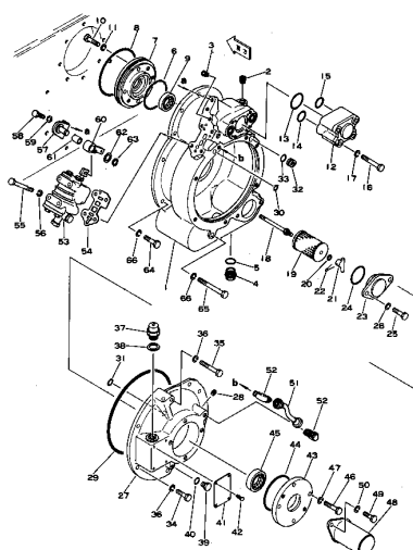
Fig. 105 P.T.O CASE
