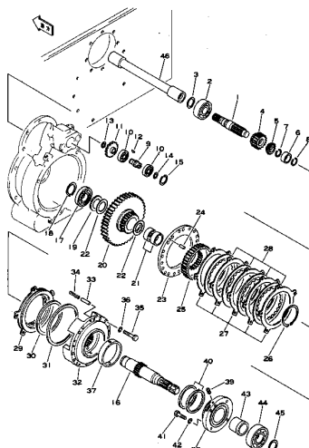
P.T.O. シフト および ギヤ Fig. 106 P.T.O SHAFT AND GEAR
