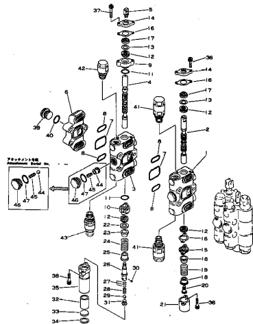
Fig. 3122 ハイドロリック コントロール バルブ (D20,21A)
