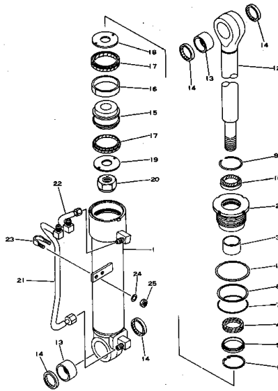
3 点 ヒッチ シリンダ Fig. 3111 3-POINT HITCH CYLINDER
