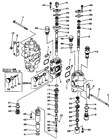
Fig. 3121 ハイドロリック コントロール バルブ HYDRAULIC CONTROL VALVE (1/3) (D20,21A)
