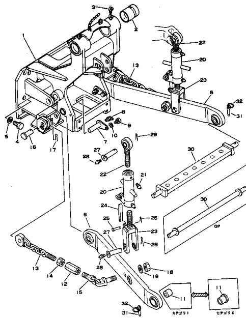
3 点 ヒッチ Fig. 201 3-POINT HITCH (1/2)
