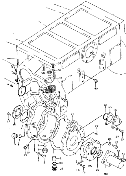
パワー テークオフ FIG.105 POWER TAKE OFF
