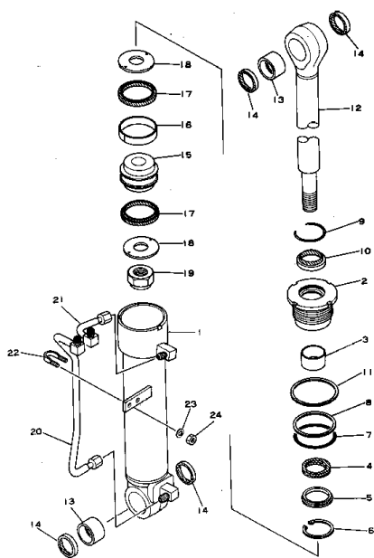
Fig. 111 3 点 ヒッチ シリンダ 3-POINT HITCH CYLINDER
