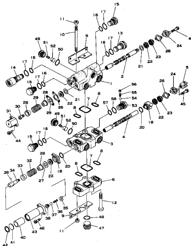
Fig. 135 ハイドロリック コントロール バルブ HYDRAULIC CONTROL VALVE
