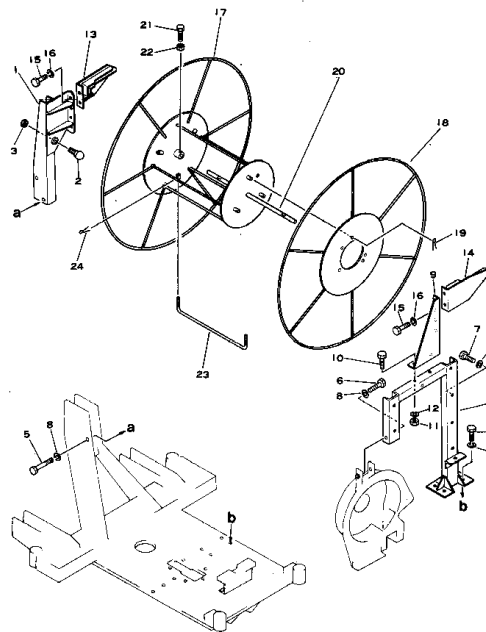
リール および ブラケット Fig. 106 REEL AND BRACKET
