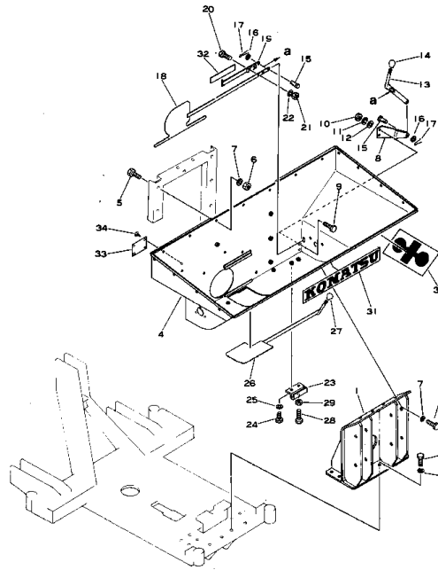
ホッパー Fig. 104 HOPPER
