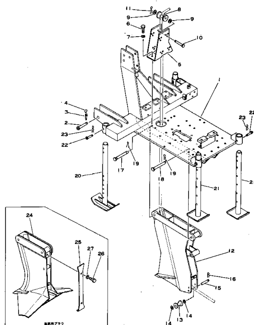
フレーム および プラウ Fig. 101 FRAME AND PLOW
