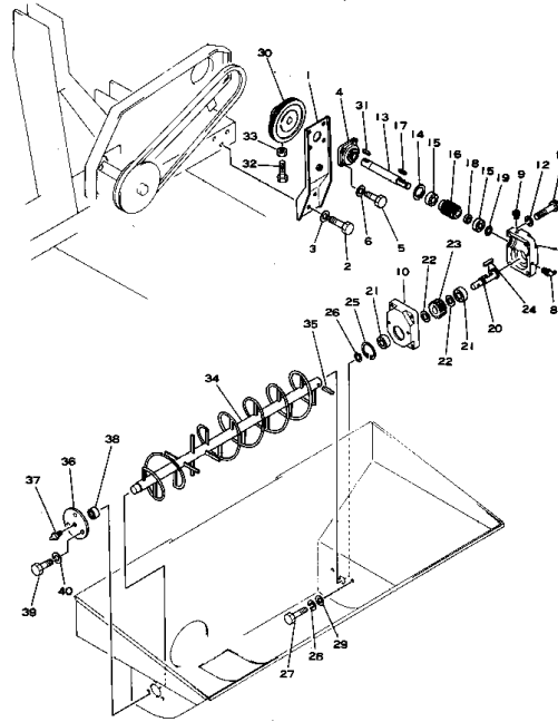
スクリーン および ギヤ Fig. 105 SCREW AND GEAR
