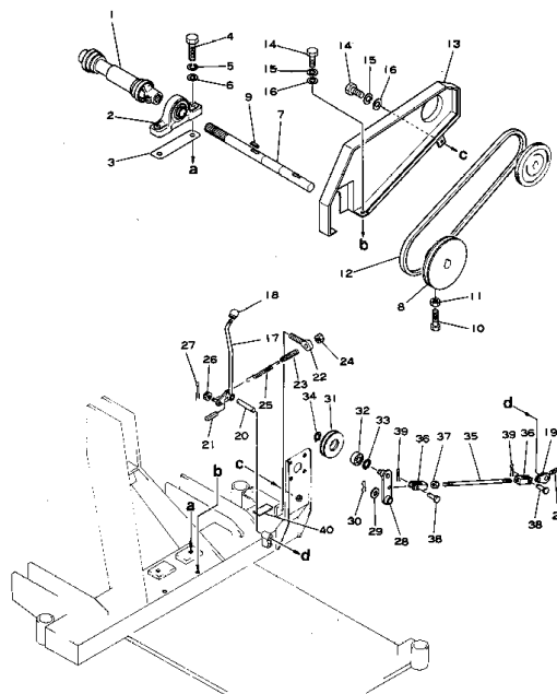
ドライブ シャフト および プーリー Fig. 102 DRIVE SHAFT AND PULLEY
