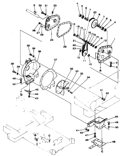
ファン および チェーン Fig. 103 FAN AND CHAIN
