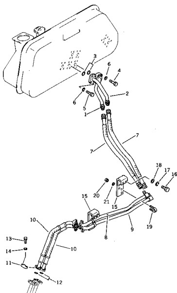
Fig. 121A ハイドロリック オイル パイピング (1/3) (適用機種 (D60, 65A Serial No. 40001~44999) (D60, 65E Serial No. 40001~44999))
