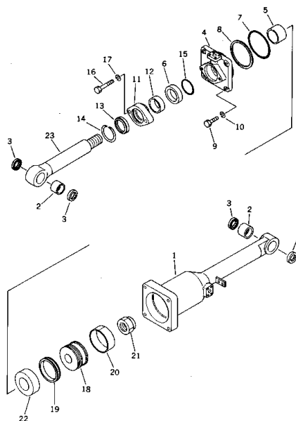
Fig. 111A チルトシリンダ (D60, 65A 適用機種) (D60, 65E 適用機種) (D60, 65E Serial No. 40001~)
