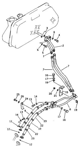
Fig. 121B ハイドロリック オイル パイピング (1/3) 適用機種 (D60, 65A Serial No. 45001~) (D60, 65E Serial No. 45001~)
