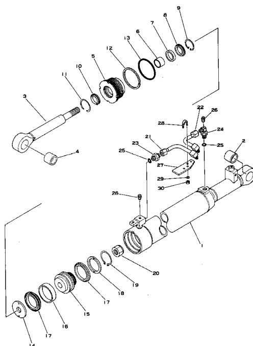
Fig. 111 チルト シリンダ TILT CYLINDER
