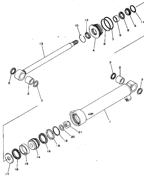
Fig. 121A ブーム シリンダ BOOM CYLINDER (DHS030-C,D,E,F,G,J,K,L,M,N,P,R,S,T,U,V,W,X,Y,Z,B1,C1,E1,G1) (適用 号 機 (Serial No. 6414-))
