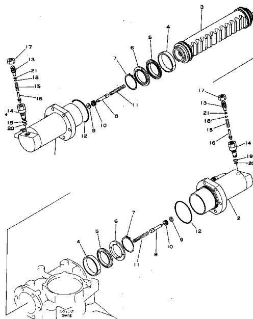
Fig. 211A スイング シリンダ SWING CYLINDER (DHS030-C,D,E,F,G,J,K,L,M,N,P,R,S,T,U,V,W,X,Y,Z,B1,C1,D1,E1,G1) (適用 機種 Serial No. 6414~)
