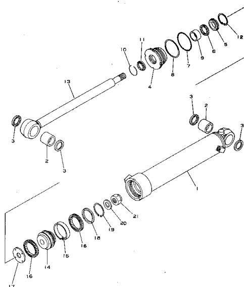
Fig. 131A アーム シリンダ ARM CYLINDER (DHS030-C,D,E,F,G,J,K,L,M,N,P,R,S,T,U,V,W,X,Y,Z,B1,C1,D1,E1,G1) (適用 号 機 (Serial No. 6414-))
