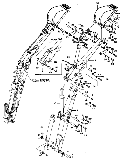
Fig. 101A BOOM (適用機種: EFGHJKLMNPQRST 15004~)
