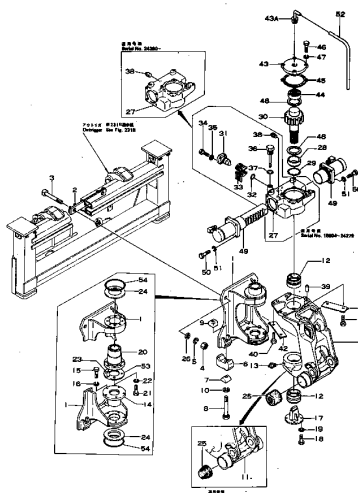
Fig. 201A SWING (適用機種 EFGHJKLMNPQRST 15004-)
