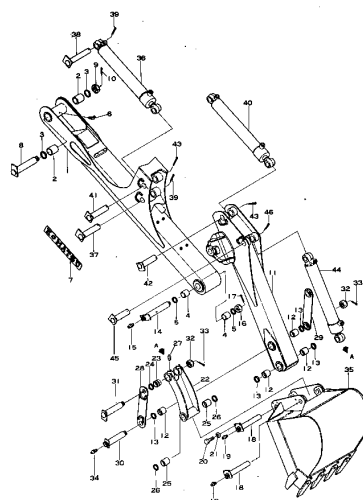
ブーム (適用号数 Fig. 101 BOOM (Serial No. ABCD 10002~14999))
