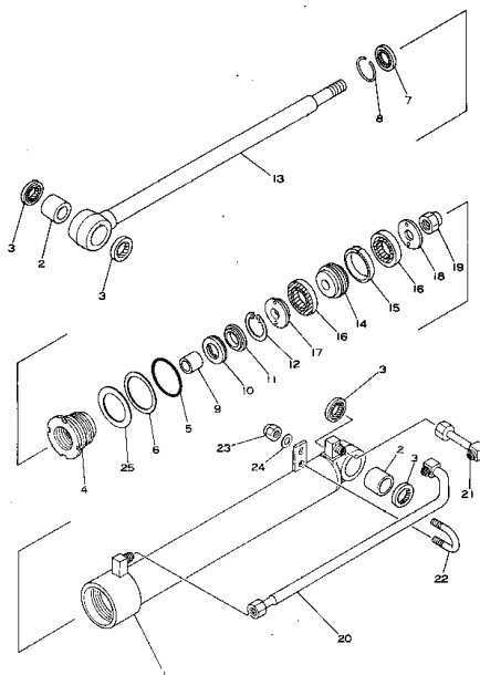
Fig. 141 バケツ シリンダ BUCKET CYLINDER
