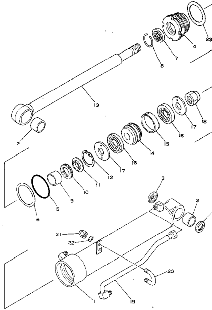
Fig. 121 ブーム シリンダ BOOM CYLINDER
