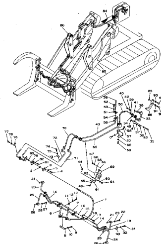
ハイドロリック・パイピング (適用号機 A 2440- ) FIG. 121A HYDRAULIC PIPING (Serial No. )
