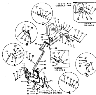
Fig. 121 ハイドロリック パイピング (適用 号機 Serial No. 1001-2439)
