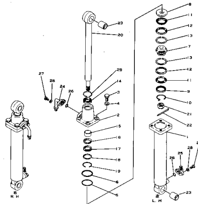
Fig. 111 ハイドラリック シリンダ (適用 号機 Serial No. 1001~ ) HYDRAULIC CYLINDER (Serial No. 1001~ )
