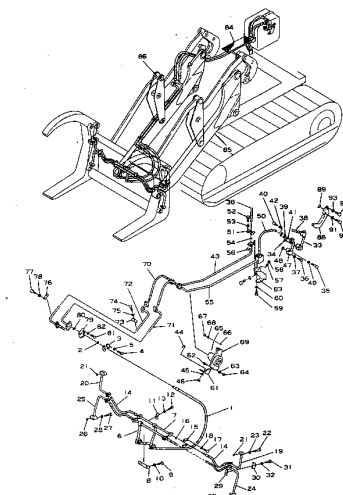
ハイドロリックパイピング (適用車種: B(2460)-(5021)) F 図. 122 HYDRAULIC PIPING (Serial No. B(2460)-(5021))
