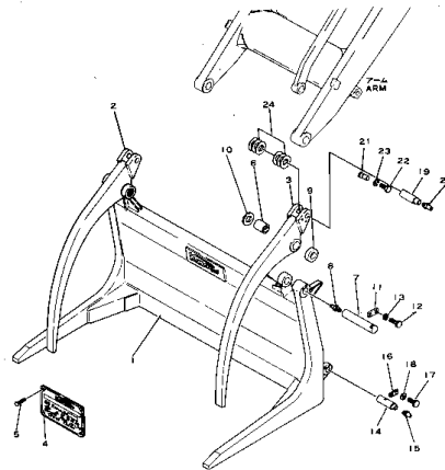
Fig. 101 スキッドローダー (適用機種 SKID LOADER (Serial No. 1001~))
