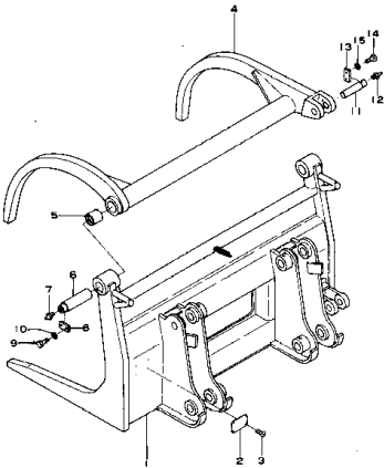
FIG. 101A スキッドローダ (適用号機 (Serial No. 81001~))
