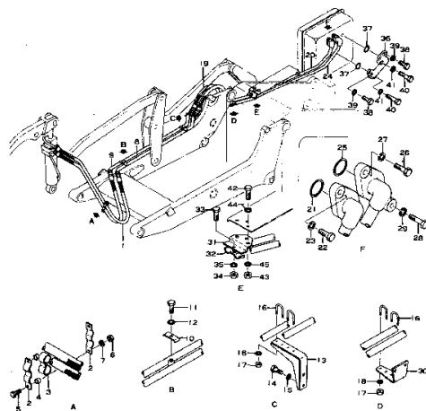
FIG. 121A PIPING (適用号機 Serial No. 81001~)
