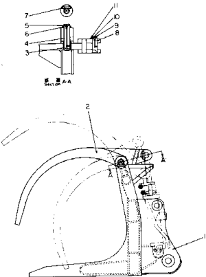
スキッドローダー (適用 号機 Serial No. A(16001~30587)) F I G. 101 SKIDLOADER
